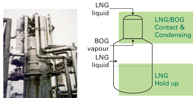
Figure 4.12 – LNG Recondenser.
